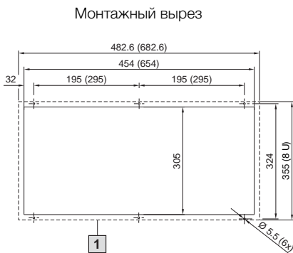
1 Опорная поверхность
