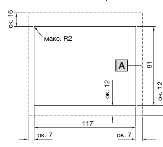
Монтажный вырез
