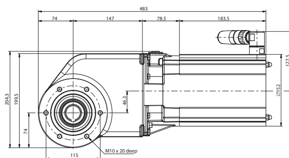
Габаритные размеры привода Danfoss VLT® OneGearDrive Hygienic®
