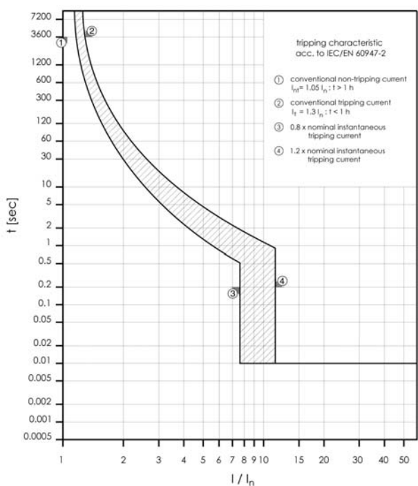
Характеристика отключения BZM1 63A, 3-пол.
