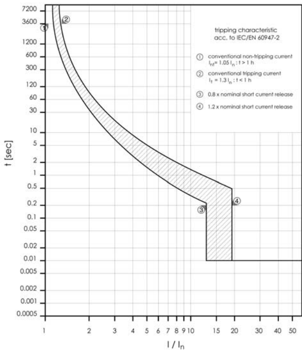
Характеристика отключения BZM1 25A, 3-пол.
