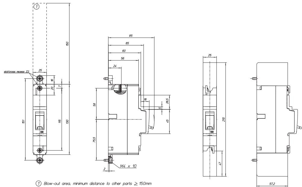
Автоматический выключатель BZM1 1-пол.
