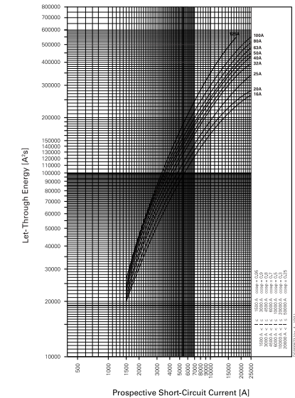
Пропускаемая энергия BZM1
