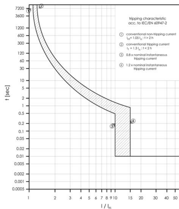
Характеристика отключения BZM1 80A, 3-пол.
