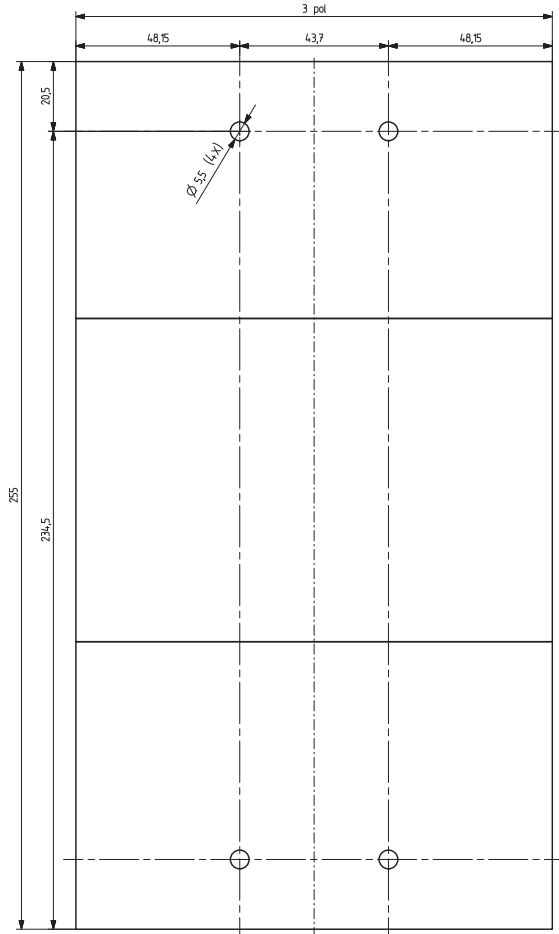
Монтажные отверстия BZM3
