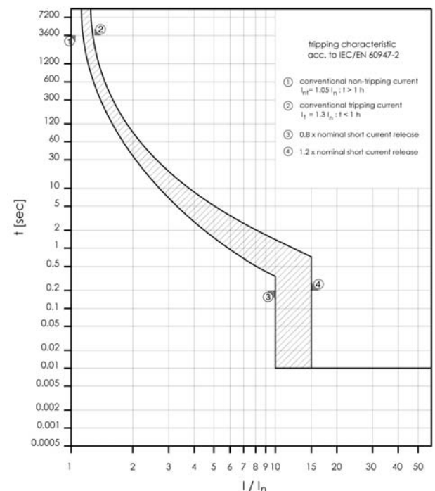
Характеристика отключения BZM1 32A, 3-пол.
