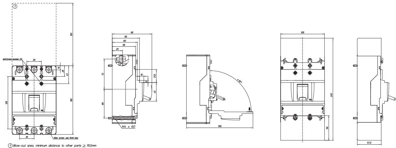
Автоматический выключатель BZM2 3-пол.
