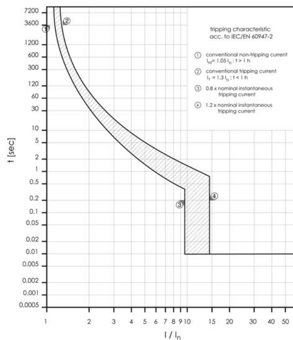
Характеристика отключения BZM1 50A, 3-пол.
