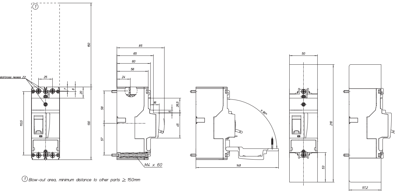
Автоматический выключатель BZM1 2-пол.
