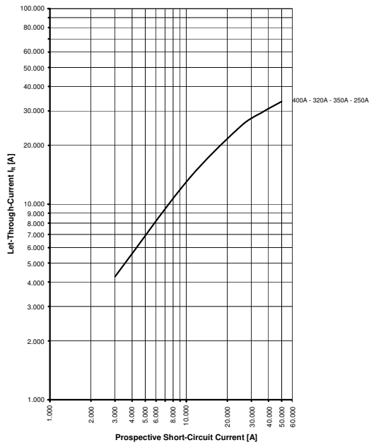
Пропускаемый ток BZM3
