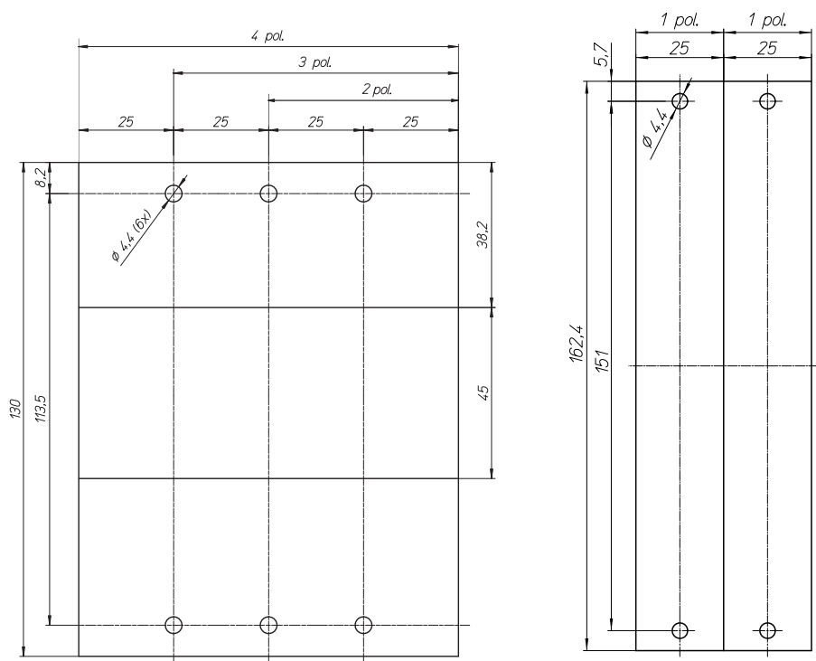
Монтажные отверстия BZM1
