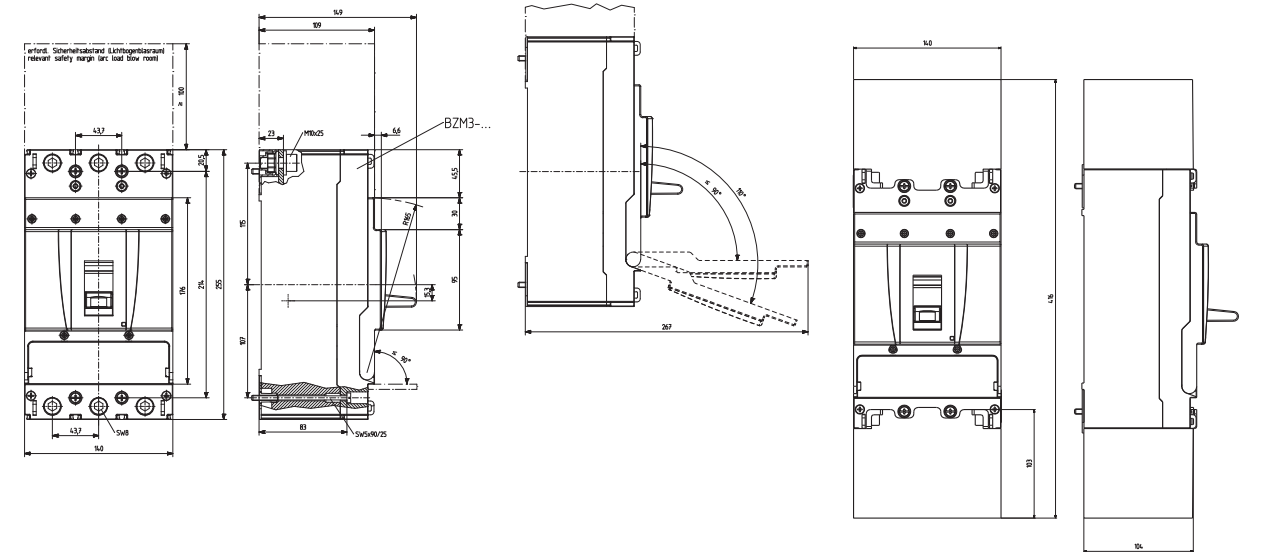
Автоматический выключатель BZM3 3-пол.
