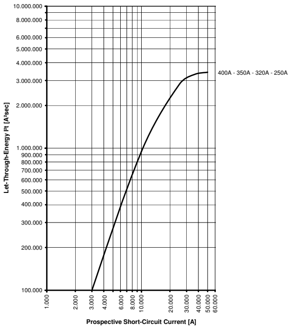
Пропускаемая энергия BZM3
