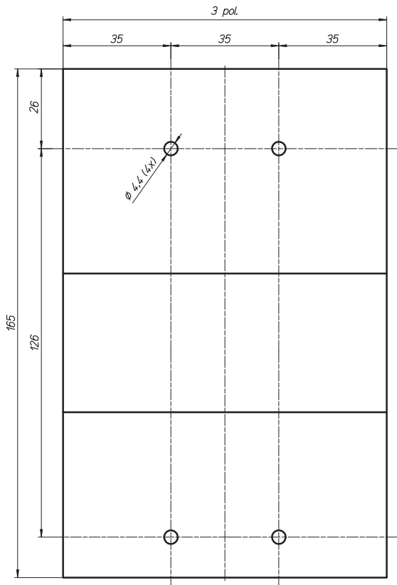
Монтажные отверстия BZM2
