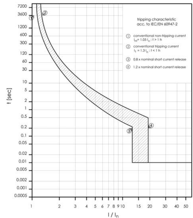
Характеристика отключения BZM1 20A, 3-пол.
