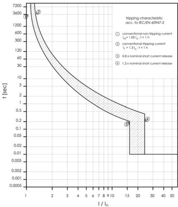
Характеристика отключения BZM1 16A, 3-пол.
