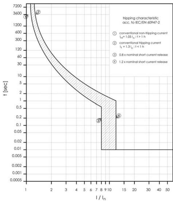
Характеристика отключения BZM1 40A, 3-пол.
