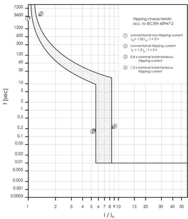
Характеристика отключения BZM2 250A
